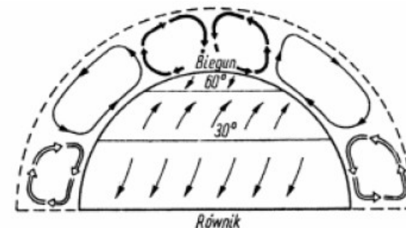
1. Schemat ogólnej cyrkulacji powietrza na półkuli północnej
