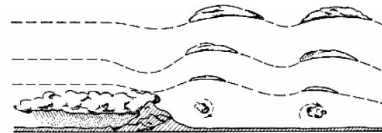
Rys. 26. Schemat zachmurzenia typu falowego (w rzeczywistości zachmurzenie może być podobne do przedstawionego schematu, ale może też od niego znacznie odbiegać)
